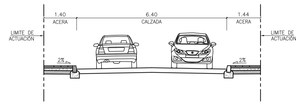
SECCION TIPO B-B' ESCALA 1/100
