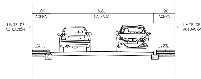
SECCION TIPO A-A' ESCALA 1/100
